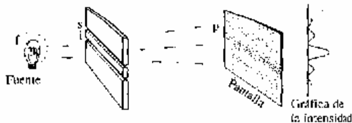
Figura 2.2. El experimento de la doble rendija, con fotones individuales de luz monocromática.
