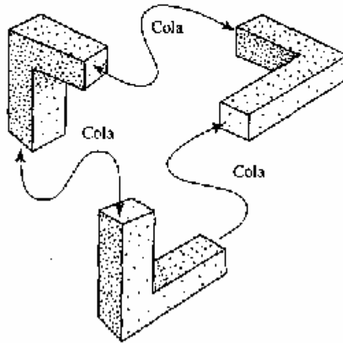
Figura 3.21 Triángulo imposible. La imposibilidad no puede localizarse; pese a todo, puede definirse en términos matemáticos precisos como una abstracción de las reglas de encolado subyacentes a su construcción.
