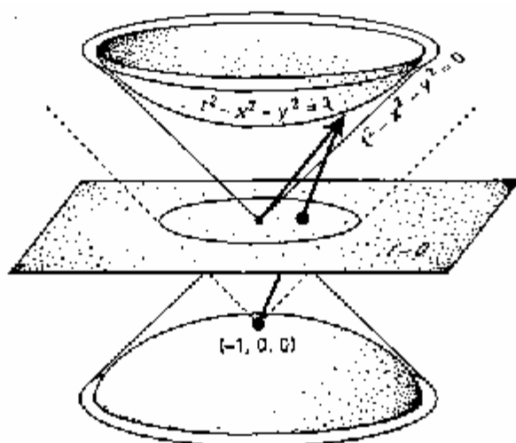
Figura 1.21. Espacio de Lobachevski insertado como una rama hiperboloide en el espacio-tiempo de Minkowski. La proyección estereográfica le hace corresponder el disco de Poincaré, cuya frontera es el círculo dibujado en el plano t = 0 .
