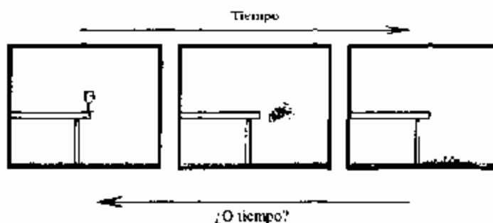
Figura 1.24. Las leyes de la mecánica son reversibles con respecto al tiempo; pese a todo, la ordenación temporal de una escena desde el fotograma derecho al izquierdo es algo que nunca se experimenta, mientras que desde el fotograma izquierdo al derecho resulta perfectamente normal.
