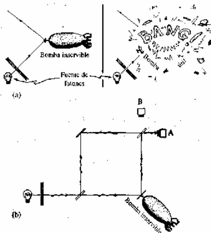
Figura 2.6. (a) El problema de la comprobación de bombas de Elitzur-Vaidman. El detonador ultrasensible de la bomba responderá al impulso de un solo fotón de luz visible –suponiendo que la bomba no es una bomba inservible debido a que su detonador está atascado–. El problema consiste en encontrar una bomba útil con garantía, dado un suministro grande de bombas dudosas. (b) El montaje para encontrar bombas útiles en presencia de bombas inservibles. En el caso de una bomba útil, el espejo inferior de la derecha actúa como aparato de medida. Cuando mide que un fotón ha seguido el otro camino, esto permite que el detector en A reciba el fotón –lo que no puede suceder en el caso de una bomba inservible–.
