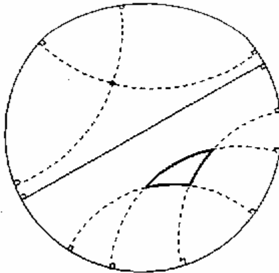
Figura 1.20. Aspectos de la geometría de un espacio de Lobachevski (hiperbólico) como el ilustrado por Limite circular I .
