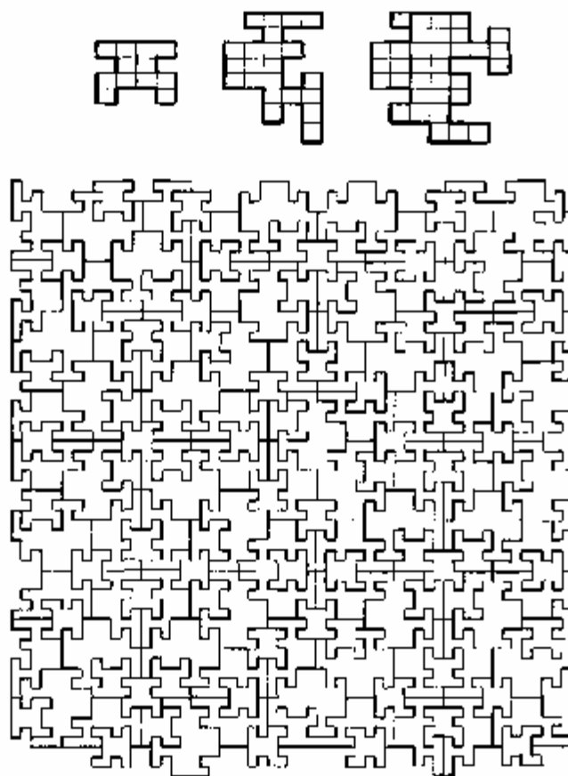
Figura 3.12. Este conjunto de tres polígonos teslará el plano solo de forma no periódica.
