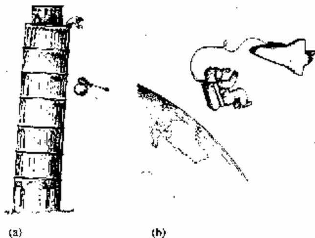
Figura 1.12. (a) Galileo arrojando dos piedras (y una videocámara) desde la Torre inclinada de Pisa. (b) El astronauta observa que el vehículo espacial se mantiene frente a él, aparentemente sin ser afectado por la gravedad.
