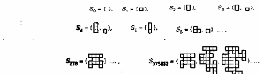
Figura 3.10. Un modelo de juguete no computable para el Universo. Los diferentes estados de este Universo de juguete determinista pero no computable están dados en términos de pares de conjuntos finitos de poliominos. Si el primer conjunto del par tesela el plano, la evolución temporal procede con un aumento del orden numérico del primer conjunto mientras que el segundo marca el tiempo . Cuando el primer conjunto no tesela el plano, los dos se permutan antes de que la evolución continúe. Sería algo así como: (S_0, S_0), (S_0, S_1), (S_1, S_1), (S_2, S_1), (S_1, S_1), (S_4, S_1), \dots, (S_{278}, S_{251}), (S_{251}, S_{278}), (S_{252}, S_{279}), \dots
