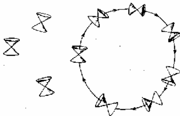
Figura 3.13. Con una inclinación suficientemente grande de los conos de luz, en el espacio-tiempo pueden darse líneas cerradas de tipo tiempo.
