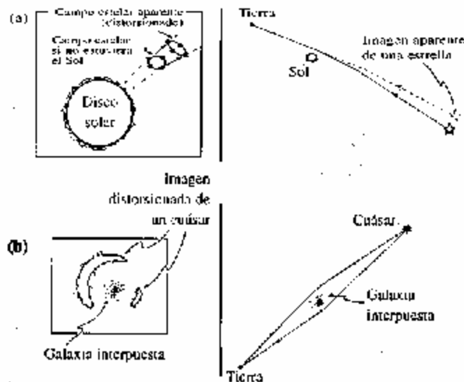
Figura 1.14. (a) Efectos observacionales directos de la gravedad sobre la luz según la relatividad general. La curvatura de Weyl del espacio-tiempo se manifiesta como una distorsión del campo estelar lejano, en este caso debida al efecto de curvatura de la luz en el campo gravitatorio del Sol. Una figura circular de estrellas se distorsionaría en una figura elíptica. (b) El efecto de curvatura de la luz de Einstein es ahora una herramienta importante en la astronomía observacional. La masa de la galaxia interpuesta puede ser estimada a partir de la medida de la distorsión que provoca en la imagen de un cuásar lejano.
