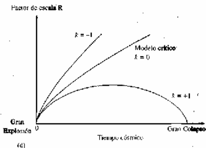
Figura 1.16 (a) Imagen espacio-temporal de un Universo en expansión con secciones espaciales euclidianas (se muestran dos dimensiones espaciales): k = 0 . (b) Como en (a), pero para un Universo en expansión (y posterior contracción) con secciones espaciales esféricas: k = +1 . (c) Como en (a) pero para un Universo en expansión con secciones espaciales de Lobachevski: k = -1 . (d) Dinámica de los tres diferentes tipos de modelos de Friedmann.
