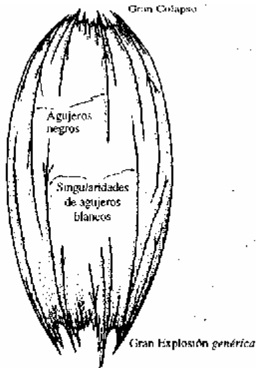
Figura 1.29. Si se elimina la ligadura Weyl = 0 , entonces tenemos también una Gran Explosión con alta entropía, con Weyl \rightarrow \infty . Un universo semejante estaría plagado de agujeros blancos, y no habría segunda ley de la termodinámica, lo que está en franca contradicción con la experiencia.
