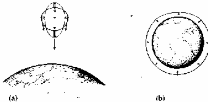
Figura 1.13. (a) El efecto de marea. Las flechas dobles muestran la aceleración relativa. (b) Cuando la esfera rodea un cuerpo material (aquí rodea la Tierra) hay una aceleración neta hacia dentro
