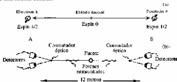
Figura 2.5. (a) Una partícula de espín 0 se desintegra en dos partículas de espín 1/2, un electrón y un positrón P. La medida del espín de una de las partículas de espín 1/2 fija de forma aparentemente instantánea el estado de espín de la otra partícula. (b) El experimento EPR de Alain Aspect y colegas. Pares de fotones son emitidos desde la fuente en un estado enmarañado. La decisión acerca de en qué dirección se mide el estado de polarización no se toma hasta que los fotones están en vuelo -demasiado tarde para enviar un mensaje al otro fotón diciéndole la dirección de medida-.
