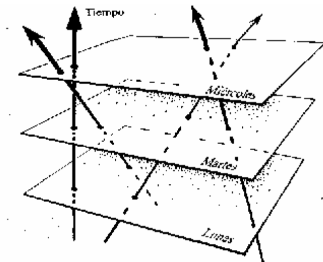
Figura 1.6. Espacio-tiempo galileano: las partículas en movimiento uniforme se representan por líneas rectas.
