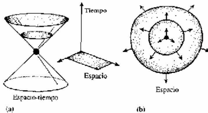
Figura 1.7 Representación de la historia de un destello luminoso en términos de su propagación en (a) el espacio-tiempo y (b) el espacio.
