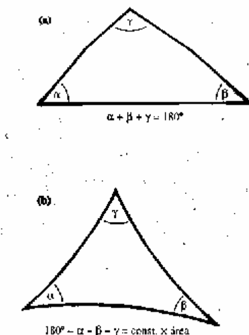
Figura 1.18 (a) Un triángulo en el espacio euclidiano. (b) Un triángulo en un espacio de Lobachevski.
