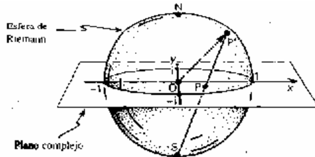
Figura 2.4. La esfera de Riemann. El punto p , que representa u = z/w en el plano complejo, es proyectado desde el polo sur s en un punto p' de la esfera. La dirección OP' , desde el centro O de la esfera, es la dirección del eje del espín para el estado superpuesto de las dos partículas de espín 1/2 .
