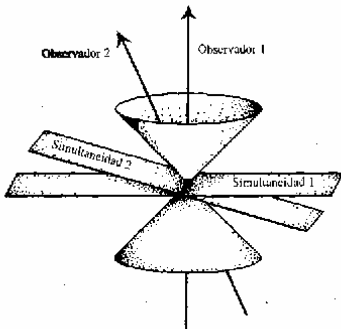
Figura 1.9. Ilustración de la relatividad de la simultaneidad según la teoría especial de la relatividad de Einstein. Los observadores 1 y 2 están en movimiento uno con respecto al otro en el espacio-tiempo. Sucesos que son simultáneos para el observador 1 no son simultáneos para el observador 2 y viceversa.
