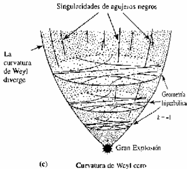
Figura 1.28. (a) La historia entera de un Universo cerrado que empieza con una Gran Explosión uniforme de baja entropía con Weyl = 0 y termina con un Gran Colapso de alta entropía que representa la coalescencia de muchos agujeros negros con Weyl \rightarrow \infty . (b) Agujero negro. (c) La historia de un Universo abierto, empezando de nuevo en una Gran Explosión uniforme de baja entropía con Weyl = 0 .
