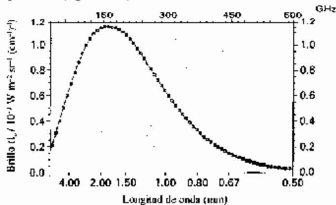
Figura 1.22. Acuerdo exacto entre las medidas de COBE del espectro de la radiación de fondo cósmico de microondas y la naturaleza térmica esperada de la radiación de la Gran Explosión (línea continua).
