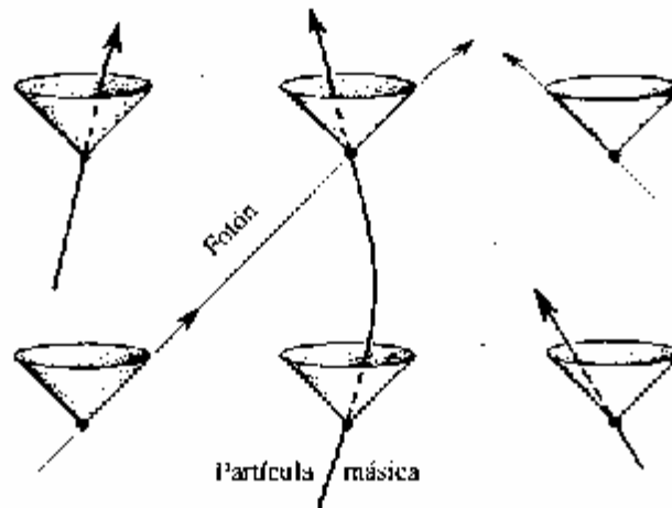
Figura 1.8. Ilustración del movimiento de una partícula en el espacio-tiempo de la relatividad especial, que se conoce como espacio-tiempo de Minkowski o geometría de Minkowski. Los conos de luz en los diferentes puntos del espacio-tiempo están alineados y las partículas solo pueden viajar en el interior de sus conos de luz futuros.
