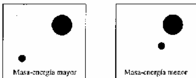
Figura 2.21. La masa-energía total de un sistema gravitante incluye contribuciones puramente gravitatorias que no son localizables.
