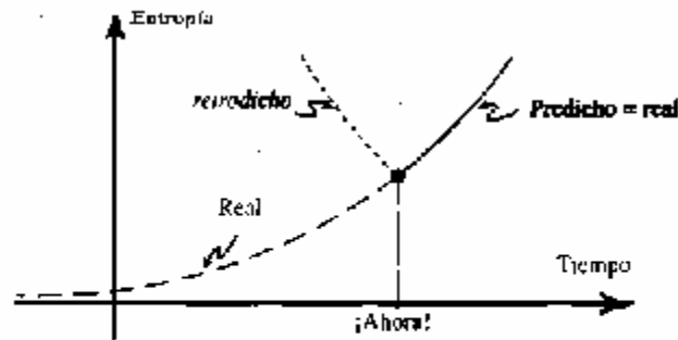
Figura 1.26. Si utilizamos el argumento representado en la figura 1.25 en el sentido contrario del tiempo, retrodecimos que la entropía también debería aumentar en el pasado, a partir de su valor actual. Esto está en franca contradicción con la observación.
