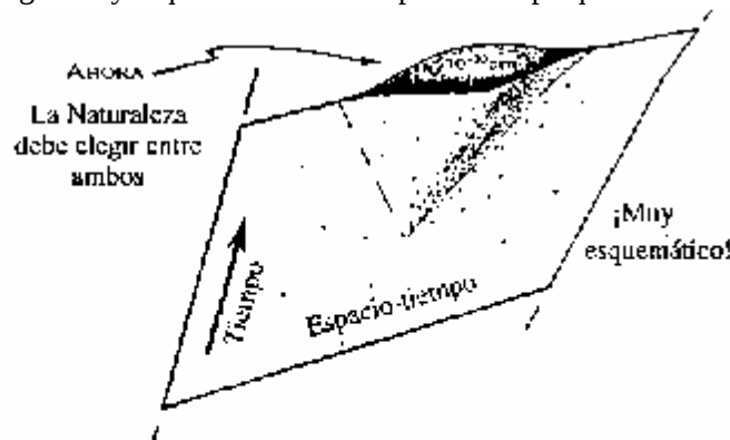
Figura 2.19. ¿Qué importancia tiene la escala de Planck de 10^{-33} cm para la reducción del estado cuántico? Idea aproximada: cuando entre los dos estados en superposición haya movimiento de masa suficiente para que los dos espacio-tiempos resultantes difieran en algo del orden de 10^{-25} cm.
