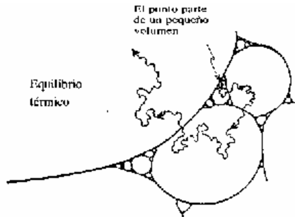
Figura 1.25. La segunda ley de la termodinámica en acción: a medida que el tiempo evoluciona, el punto en el espacio de fases entra en compartimentos de volumen cada vez mayor. En consecuencia, la entropía aumenta continuamente.
